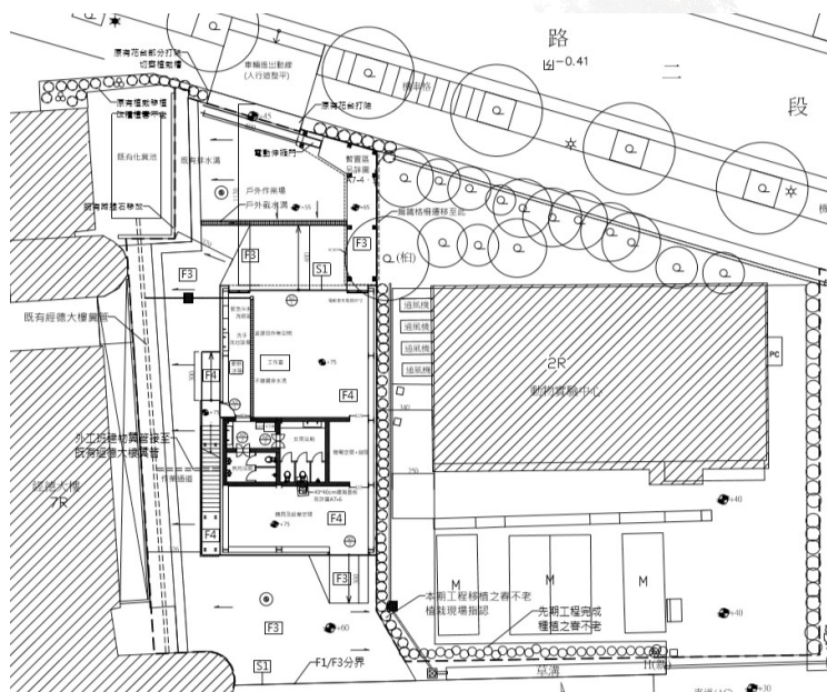
資源回收場環境整備及外工班遷建配置圖（執行中）
